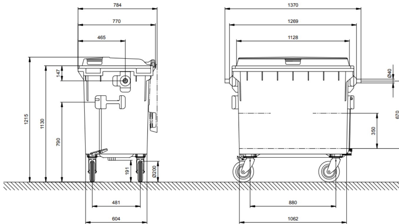
Müllbehälter MGB 660 L
