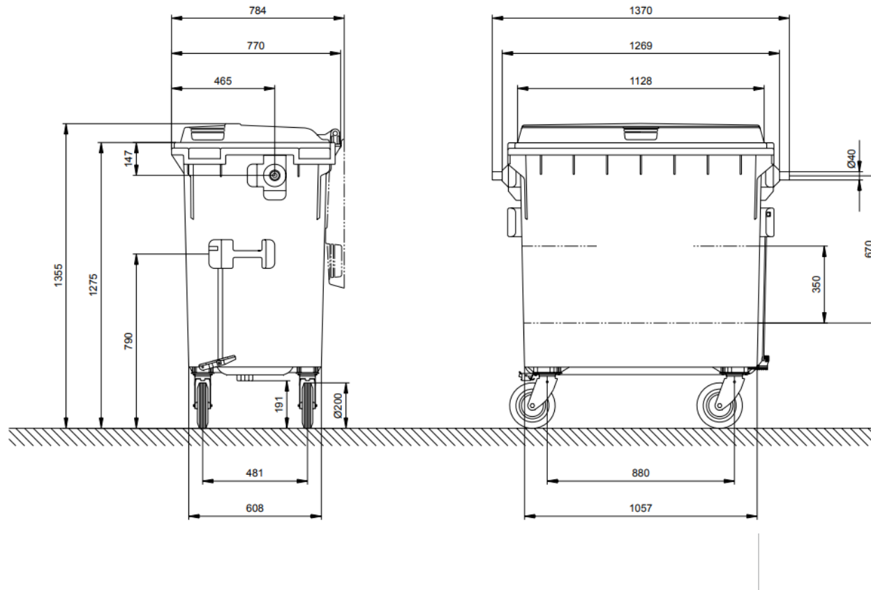
Abfallbehälter MGB 770 L
